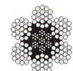
6×25 ( Fi ) +IWRC
