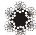
6×26 ( WS ) +FC
