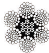
6×36 ( W S ) +IWRC
