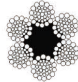
6×36 ( W S ) +FC
